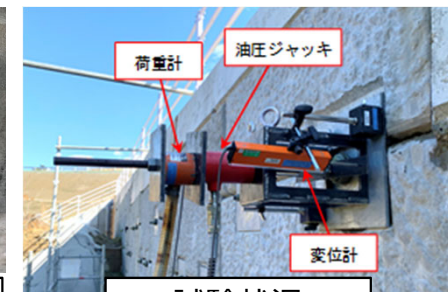
試験状況
