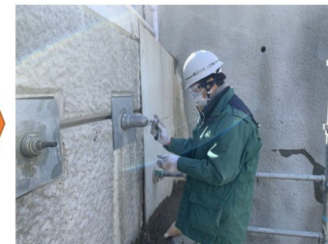
（施工後）頭部キャップ取付け （防錆剤を含む）
