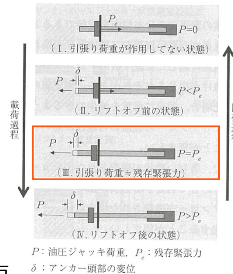
リフトオフ荷重の定義
