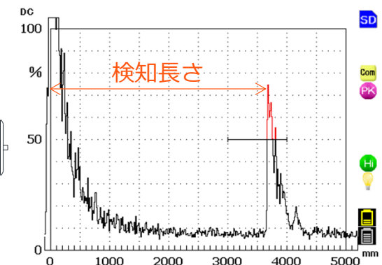
観測波形例 (補強材端部を検知)
